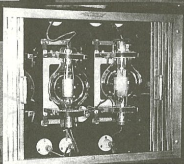
初期の真空管式長波送信機（1929年頃）
