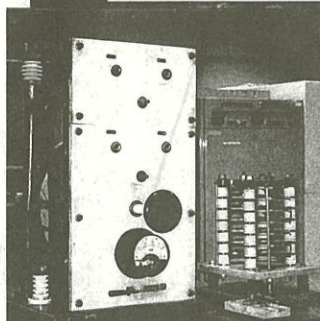
原始的送信機（テスラコイルと放電電極）
